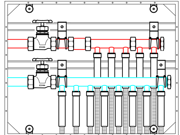
PARTICOLARE COLLETTORE SANITARIO
